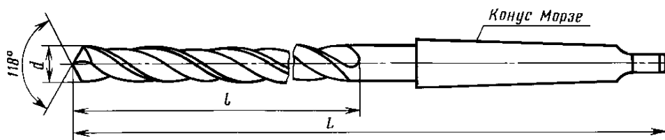
Вариант исполнения сверл с шейкой
